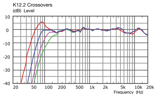
Réponse en fréquence dans l'axe de la K12.2 :
