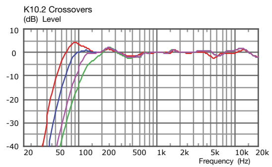
Réponse en fréquence dans l'axe de la K10.2 :
